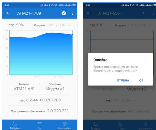
Рис. 3.4 Создание Bluetooth-соединения с модемом ATM: а) – соединение установлено; б) – соединение установить не удалось
