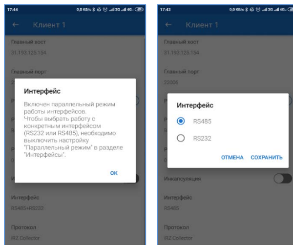
Рис. 3.28 Выбрать интерфейс для соединения типа Клиент : а) – выбрать интерфейс невозможно: включен параллельный режим работы интерфейсов; б) – RS485 или RS232
