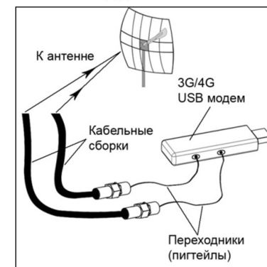
Пример подключения 3G/4G USB модема
