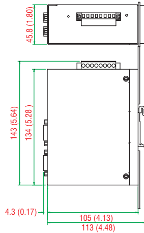
NPort IA5450A NPort IA5450AI
