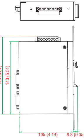
NPort IA5150A NPort IA5150AI NPort IA5250A NPort IA5250AI
